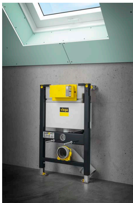
Til lave monteringshøjder: det 820 mm høje wc-element
