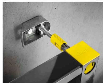
Prevista Dry vægbeslag: dybdeindstilling uden værktøj
