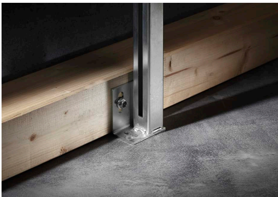
Prevista Dry montering: montering af foden.
