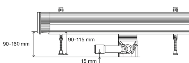
Også variabel i højden: Monteringshøjde mellem 90 og 165 mm.
