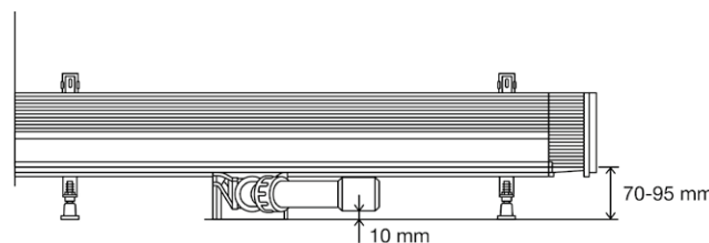
Ekstrem lav: Det specielle afløb til renovering reducerer monteringshøjden til 70 mm.
